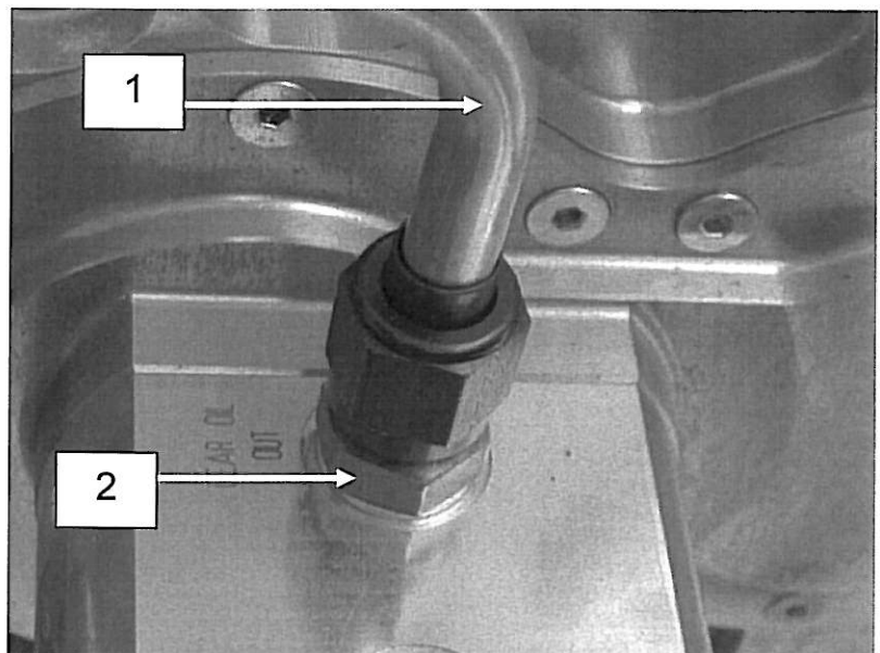
Bild 1 Aluminiumrohrleitung / Fig. 1 Pipe connection
