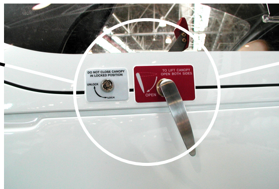
Left Side - Exterior Canopy Frame
